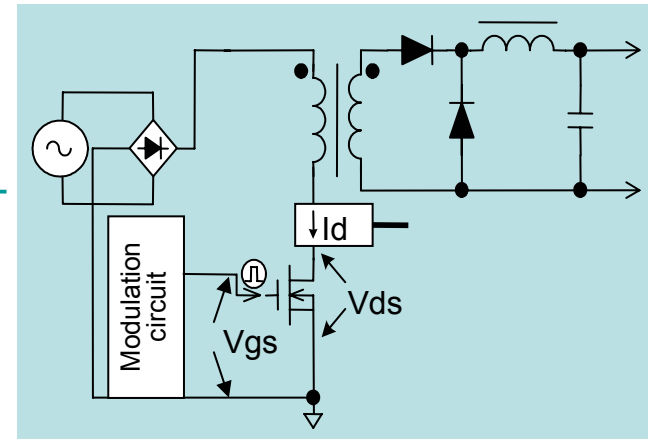
Prinzipialschaltung mit Messpunkten
