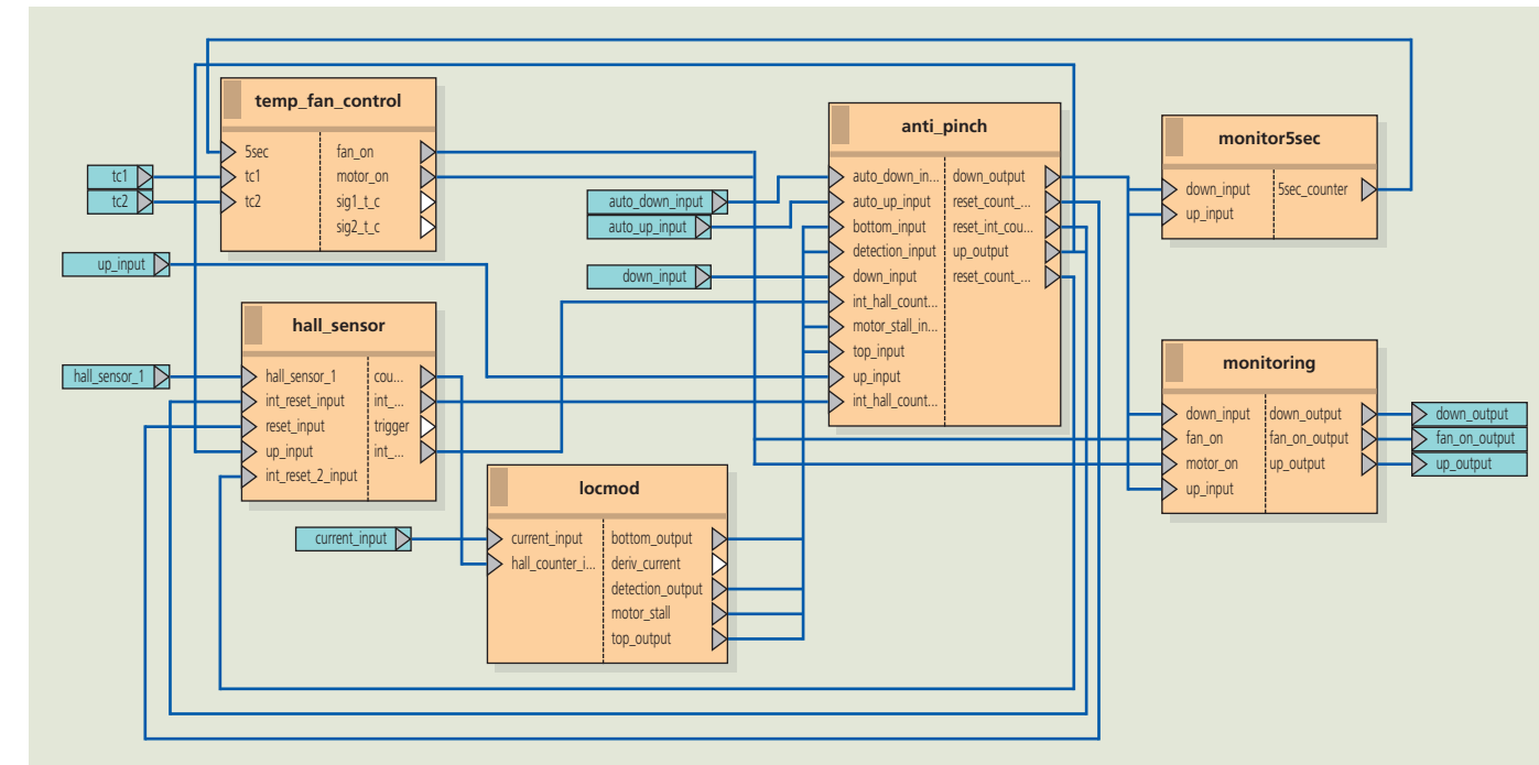
Bild 3: INTECRIO-Blockdiagramm des Steuerungs-/Regelungssystems für die Einklemmsperre.
